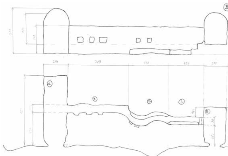
b) alaprajza és oldalnézetei (saját rajz)
