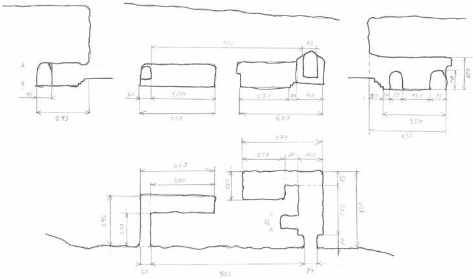
A C.) bunker alaprajza és oldalnézetei (saját rajz)
