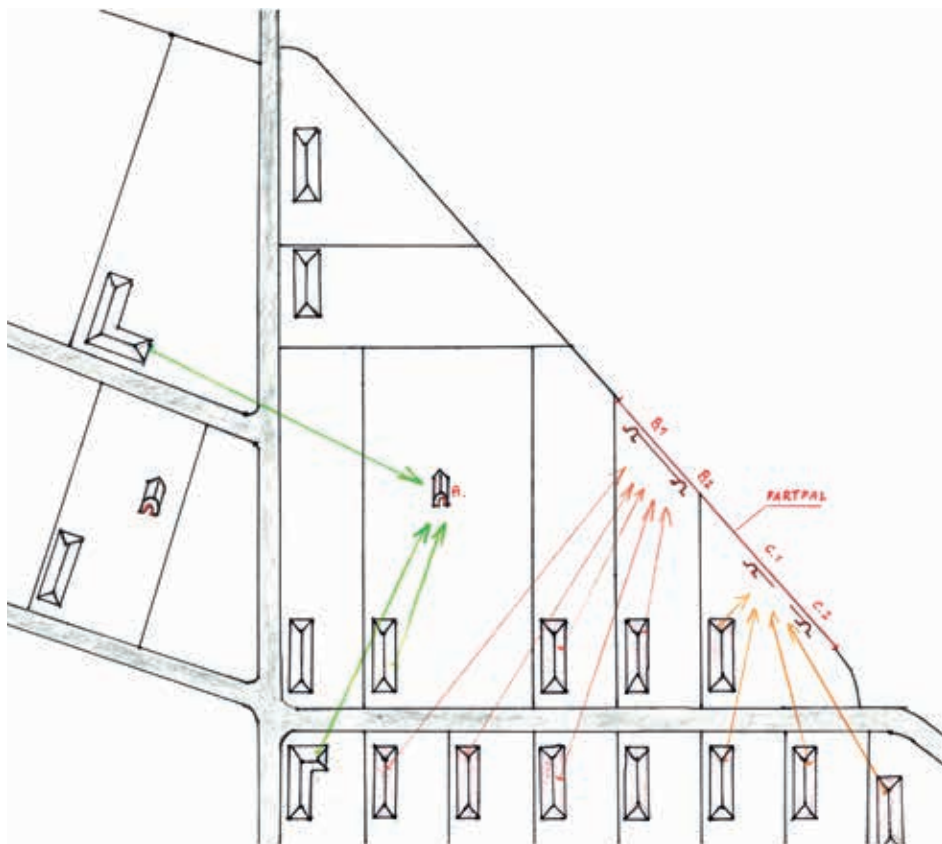
Farnad, Tyekó utca alaprajza, evakuációs terv (Forrás: Vrábel Lenke)
