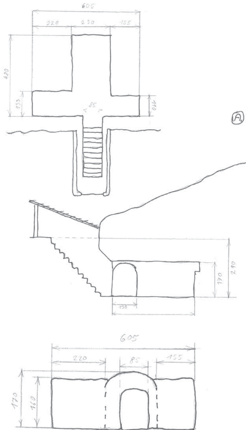
Az A) bunker alaprajza és oldalnézetei (saját rajz)
